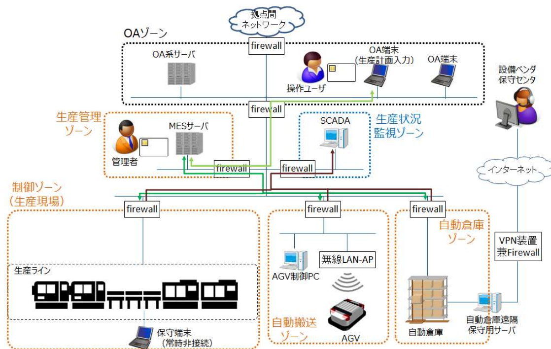
図 5-4 要件に対する各ゾーンでの対策例
