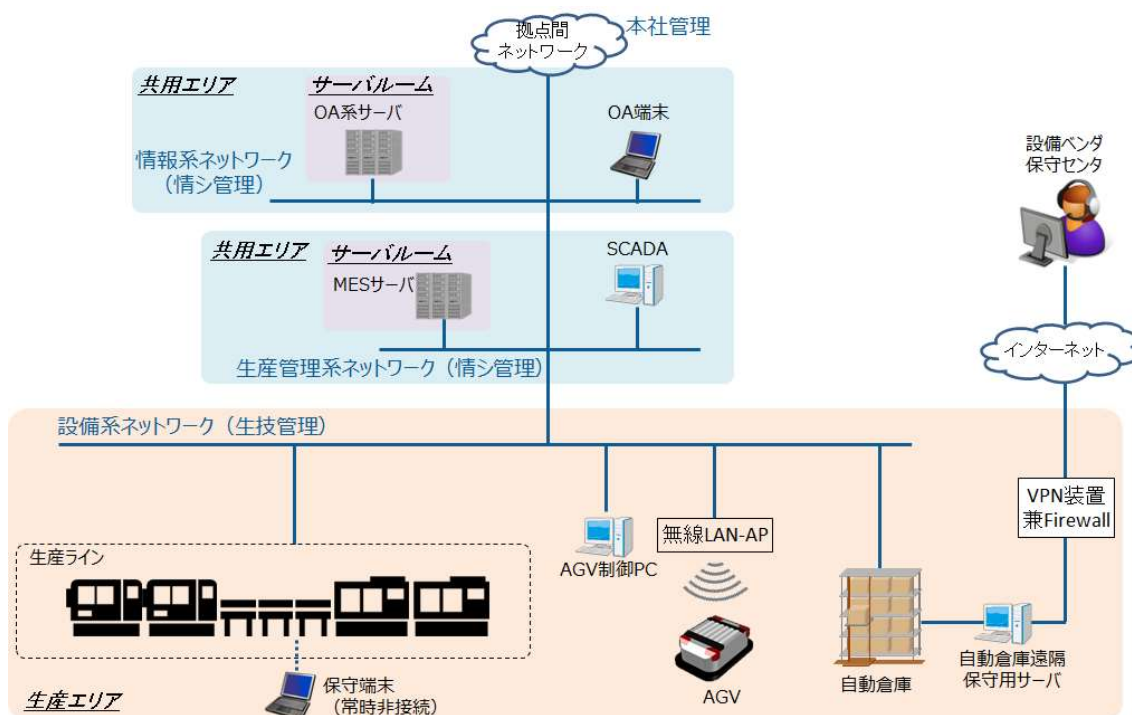
図 5-1 3章のFAシステム構成例(再掲)
